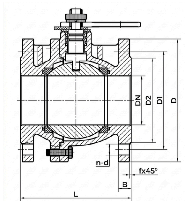
DN50-DN80
