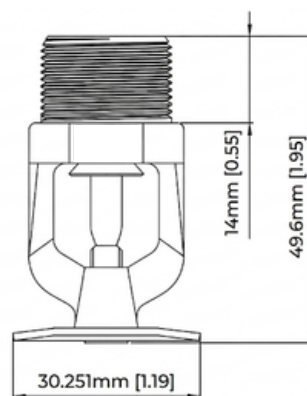
Pendent Sprinkler
